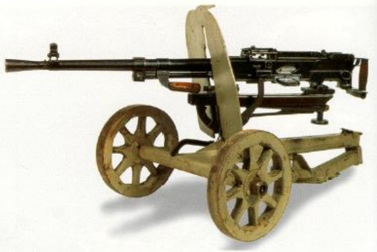
СГ-43, станковый пулемет Горюнова образца 1943 г.
